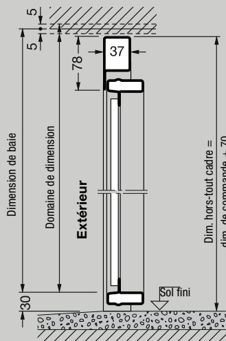
Coupe verticale
