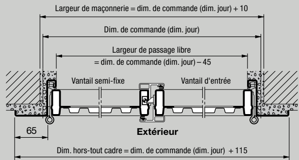
Coupe horizontale
