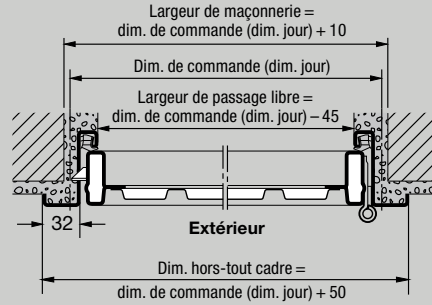
Coupe horizontale
